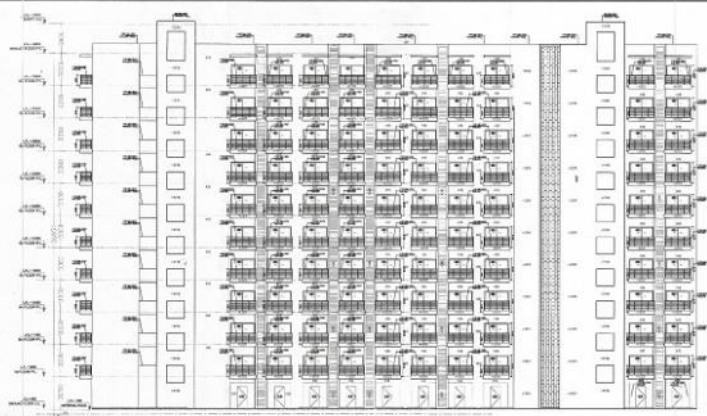
ELEVATION A
