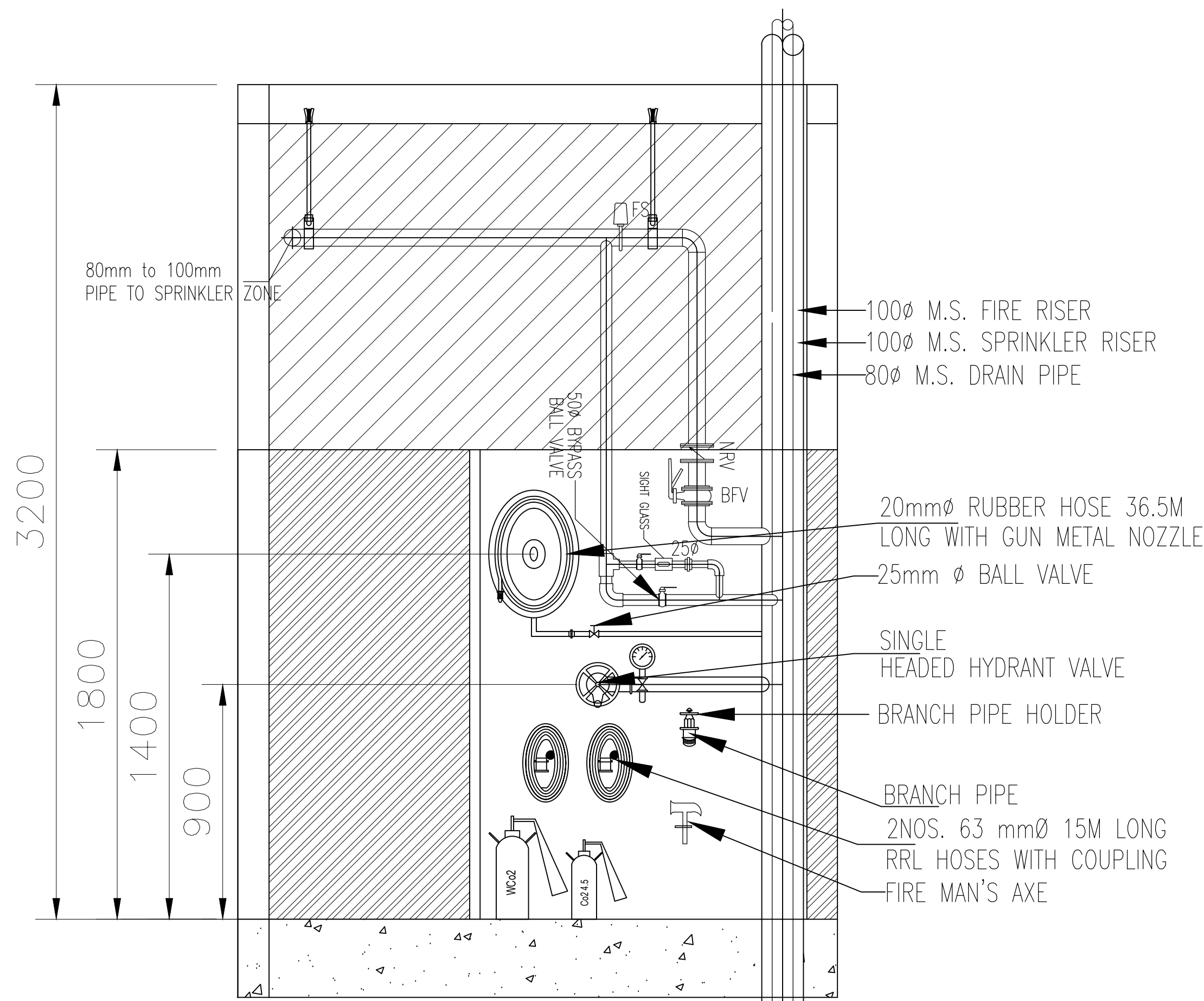
ELEVATION TYP. FHC
