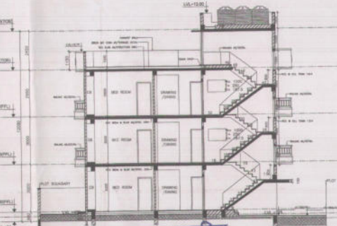
SECTION AA मानचित्र विकास प्राधिकरण
