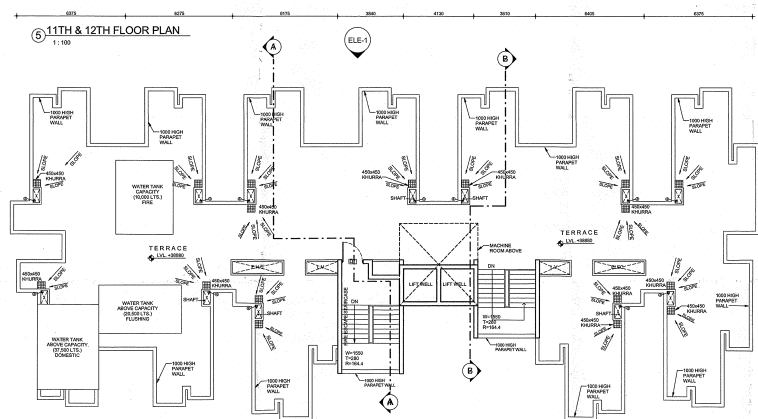
6 TERRACE PLAN 1:100
