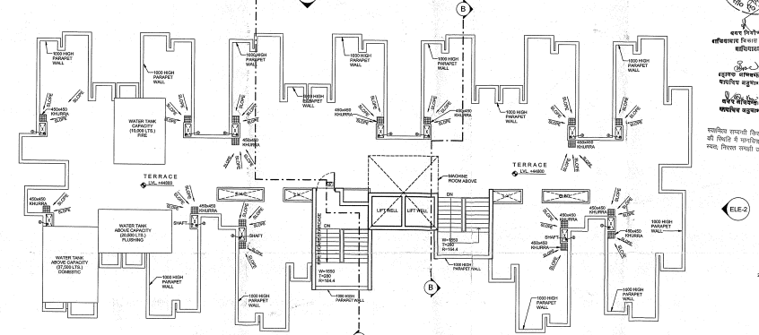
⑥ TERRACE PLAN 1:100
