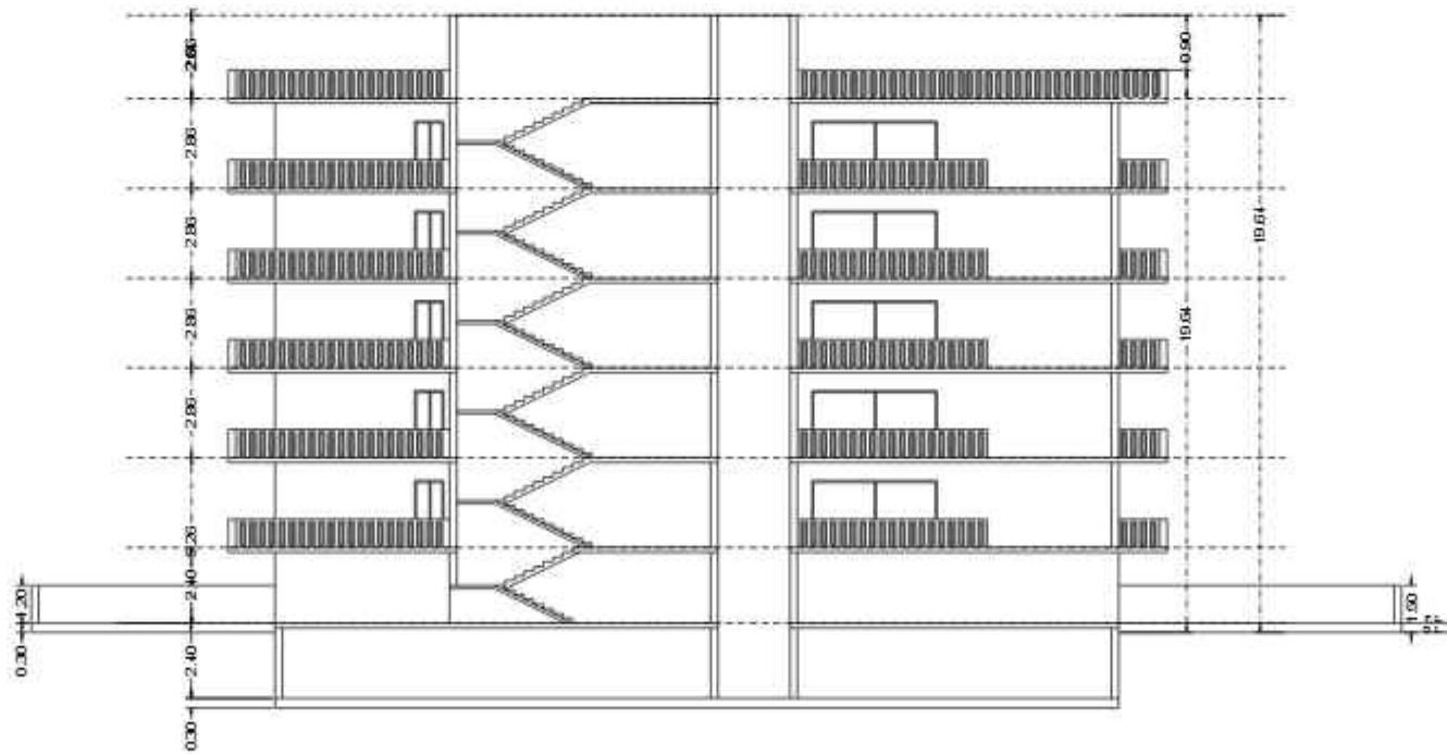
SECTION A-B
