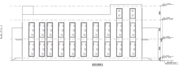
ELEVATION 4 SCALE=1:100
