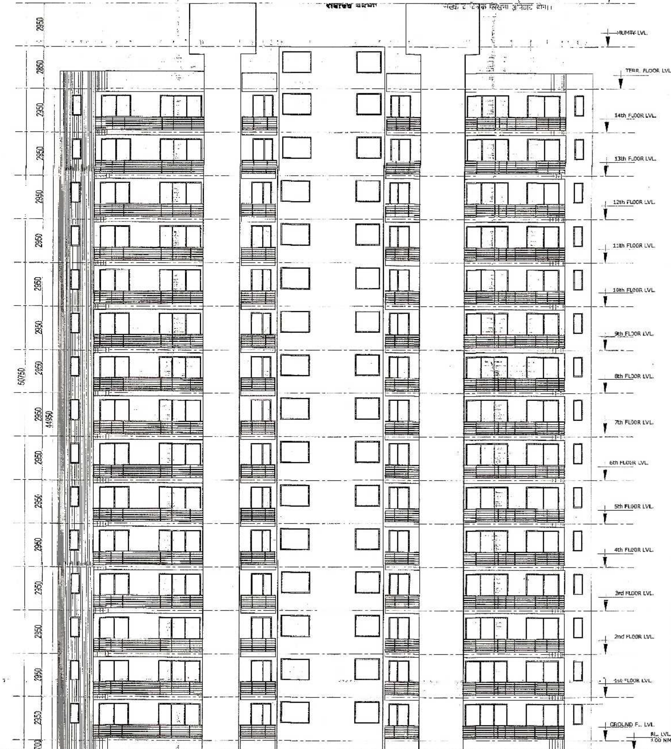
ELEVATION
