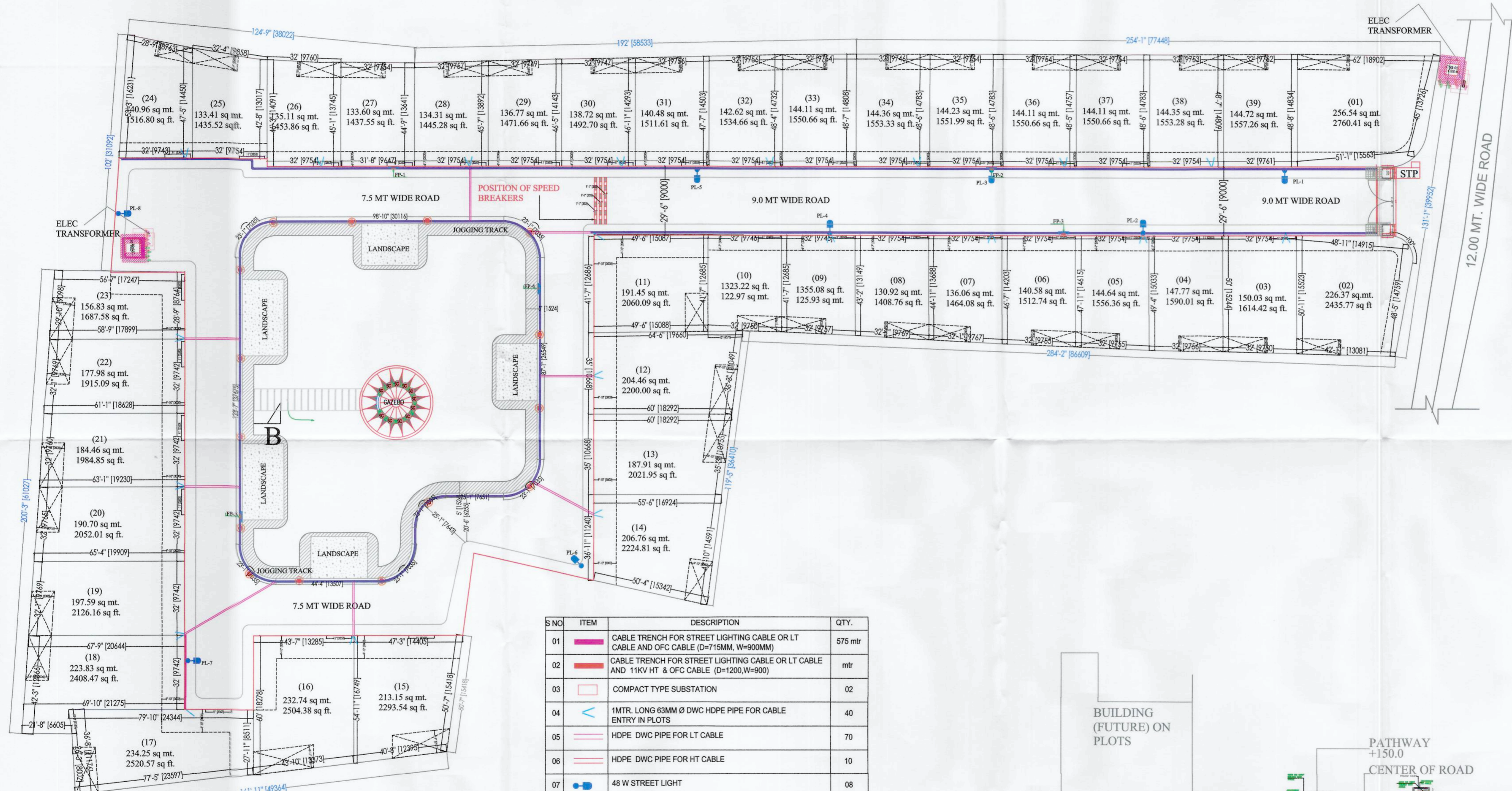
LAYOUT MAP Scale: 1"=8'-0"
