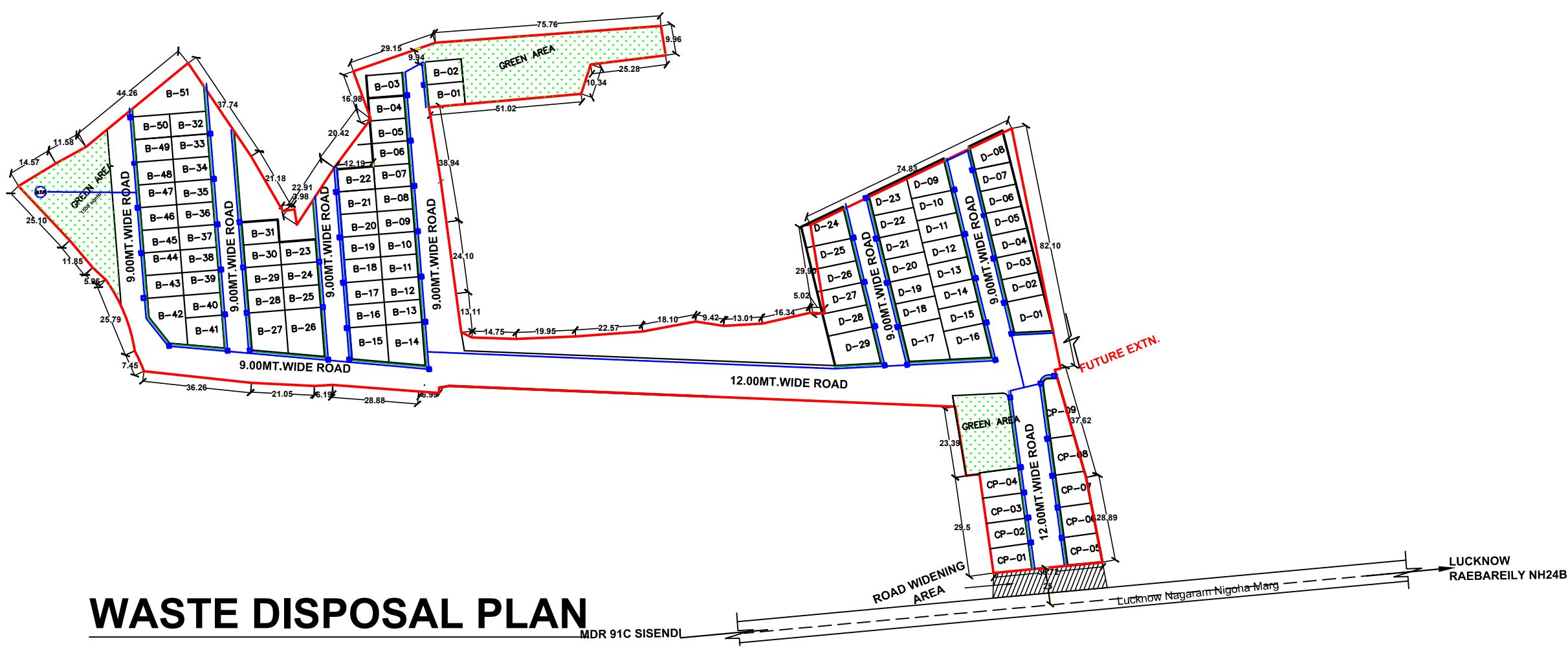
WASTE DISPOSAL PLAN SCALE: 1:100
