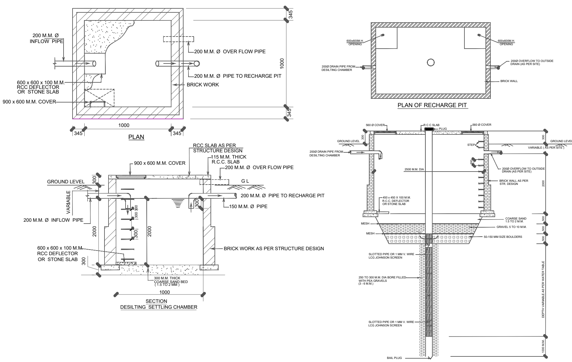
WATER RECHARGING PIT SCALE: (N.T.S.)
