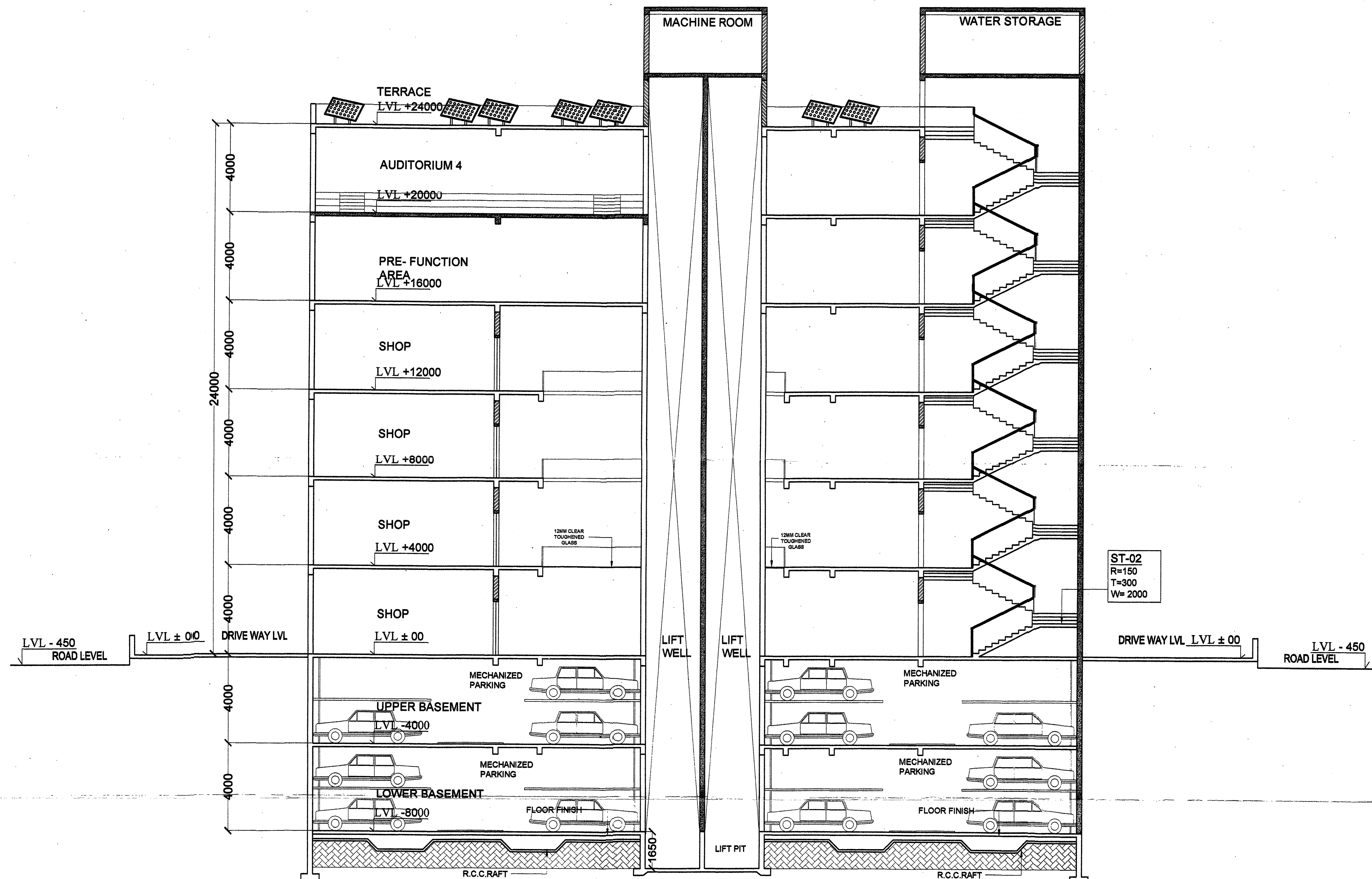
SECTION A-A'
